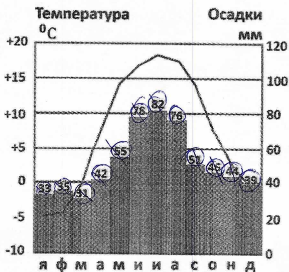
Климатограмма г. Брест
